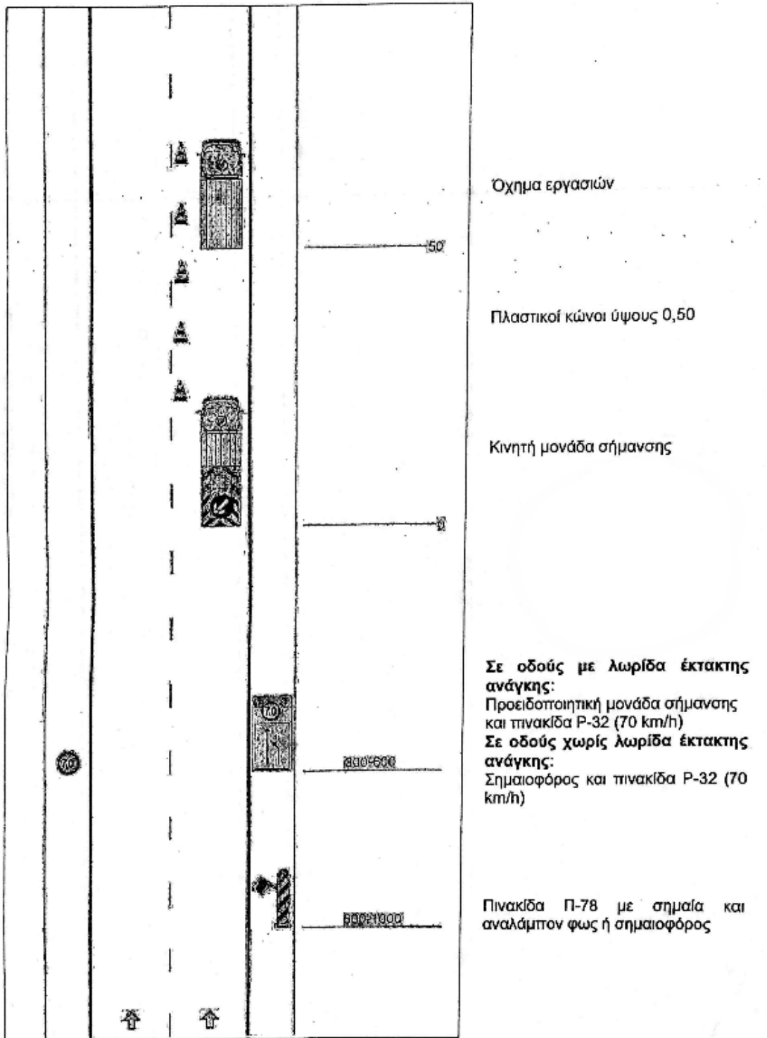
ΣΧΕΔΙΟ 3 : Σήμανση εκτελούμενων εργασιών μικρής διάρκειας στη δεξιά λωρίδα κυκλοφορίας σε οδό με διαχωριστική νησίδα (διαστάσεις σε m)
