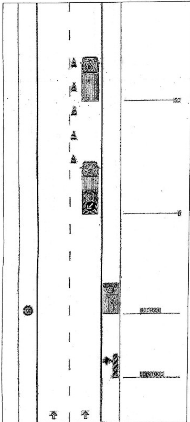
ΣΧΕΔΙΟ 3 : Σήμανση εκτελούμενων εργασιών μικρής διάρκειας στη δεξιά λωρίδα κυκλοφορίας σε οδό με διαχωριστική νησίδα (διαστάσεις σε m)
